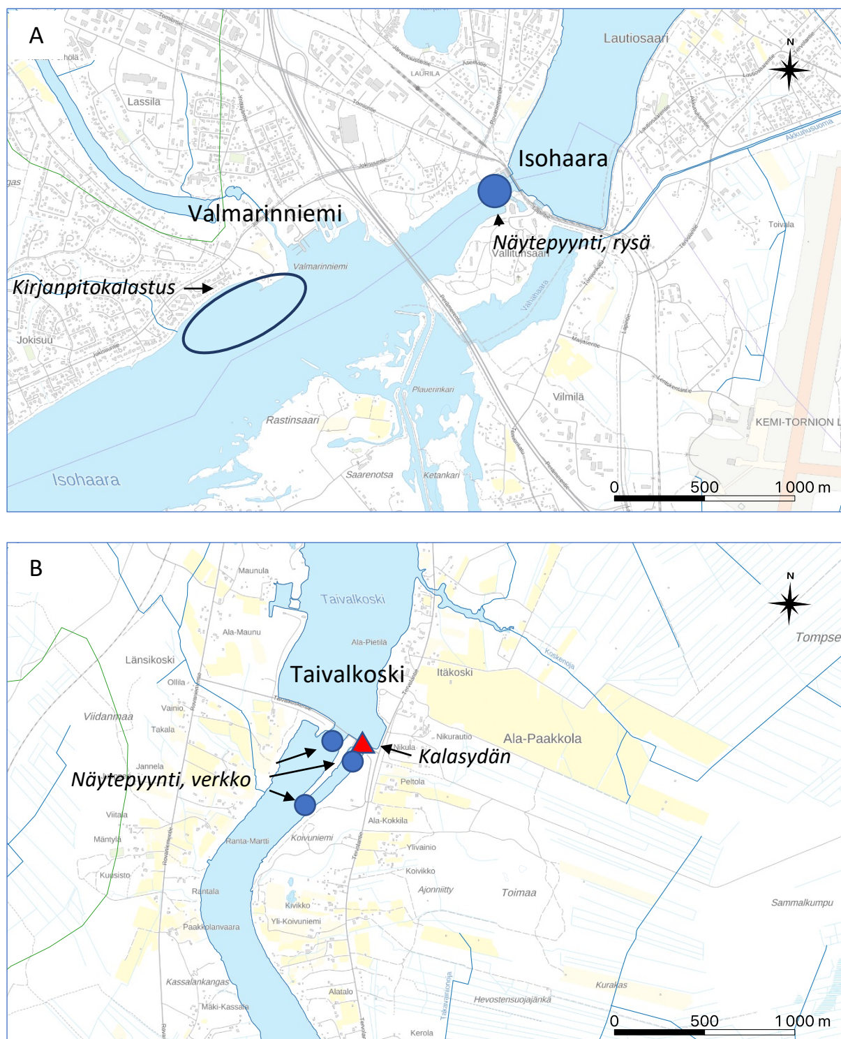
Kuva L1. Näytepyynnin ja kirjapitokalastuksen näytteenottoalueet Isohaaran voimalaitoksen alapuolella (A) sekä näytepyynnin näytteenottoalue Taivalkosken voimalaitoksen alapuolella ja Kalasydämen sijainti (B) vuonna 2021. (Kapsi-taustakartta: Maanmittauslaitos 2021, CC-BY-4.0 via kartat.kapsi.fi.)
