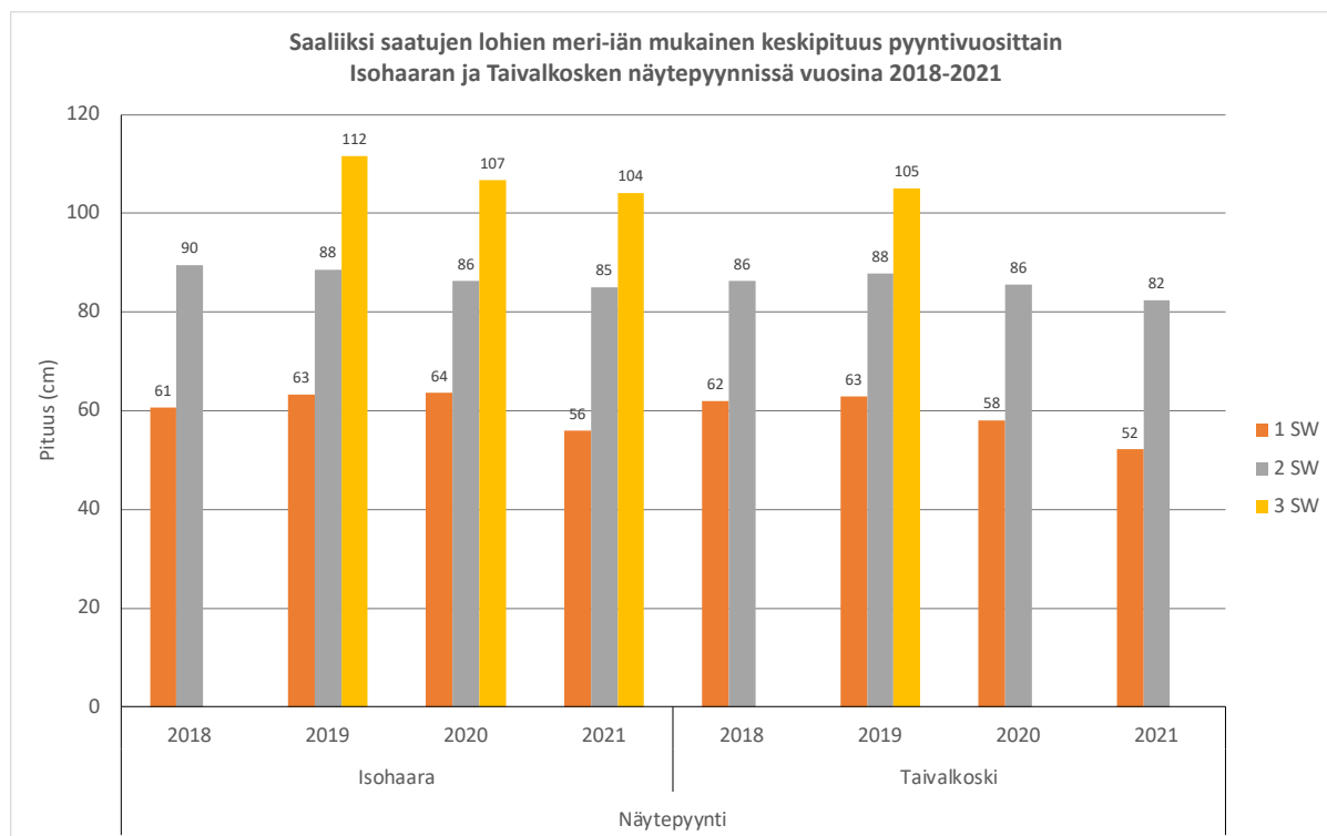
Kuva 5. Lohien meri-ikä mukainen keskipituus pyyntivuositain Isohaaran ja Taivalkosken alapuolen näytepyynnissä vuosina 2018–2021 (1 SW = yksi merivuosi, 2 SW = kaksi merivuotta, jne.). Kaavion pylväisiin merkityt luvut kuvaavat meri-ikäkohtaista keskipituutta (cm).
